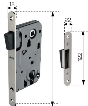
ZAMEK NIKEL LOCK NICKEL
