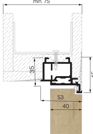
ZABUDOWA G-K / DRYWALL min. 75
