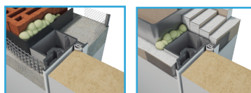
MOŻLIWE WYKOŃCZENIA OŚCIEŻNICY POSSIBLE DOOR FRAME FINISHES
