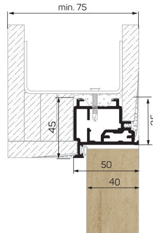
ZABUDOWA G-K / DRYWALL min. 75
