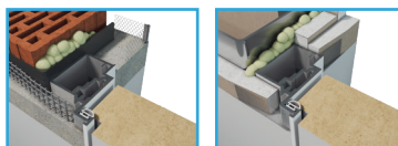
ZEWNĘTRZNA - ZABUDOWA MUR/G-K EXTERNAL - BRICK/DRYWALL
