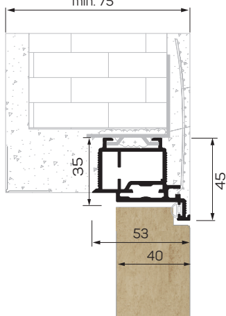
ZABUDOWA MUR / BRICK WALL min. 75
