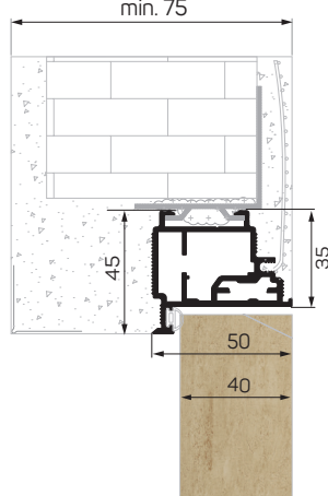
ZABUDOWA MUR / BRICK WALL min. 75
