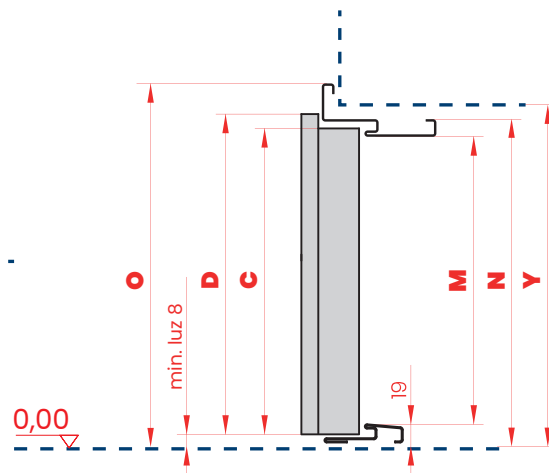
PRZEKRÓJ PIONOWY
