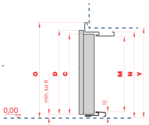
PRZEKRÓJ PIONOWY
