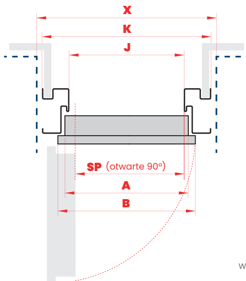
PRZEKRÓJ POZIOMY
