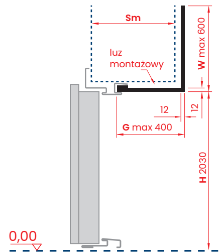
PRZEKRÓJ PIONOWY
