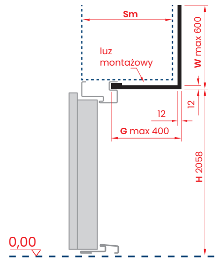
PRZEKRÓJ PIONOWY
