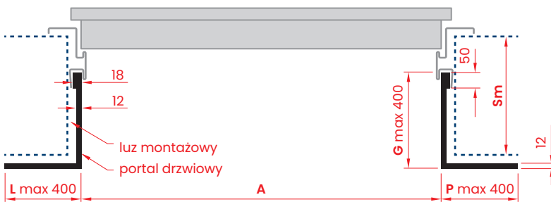
PRZEKRÓJ POZIOMY
