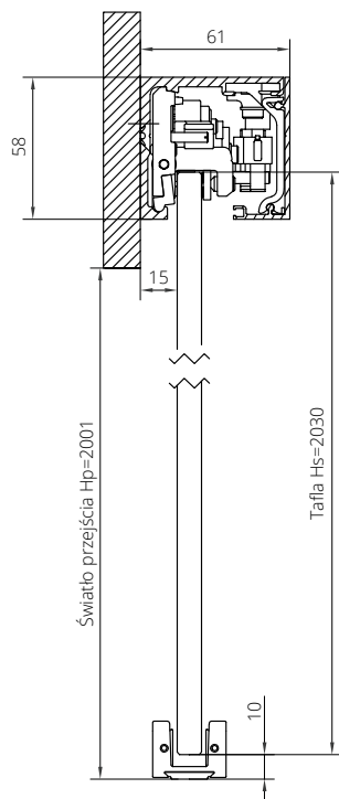
Drzwi z pochwytem podłużnym
