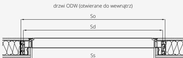
drzwi ODW (otwierane do wewnątrz)
