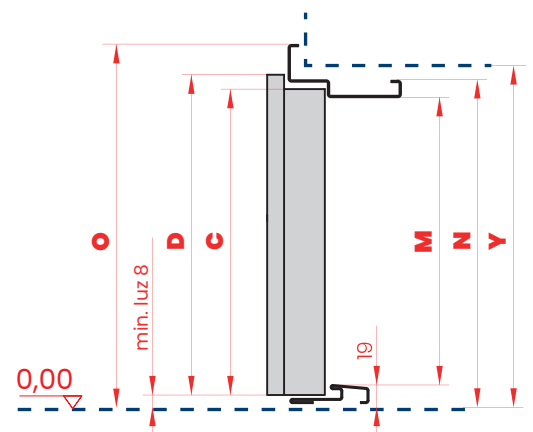
PRZEKRÓJ PIONOWY
