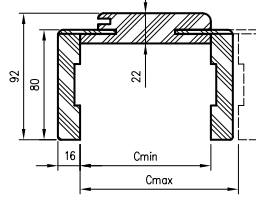
Przekrój OR/ORC z ką. T80
